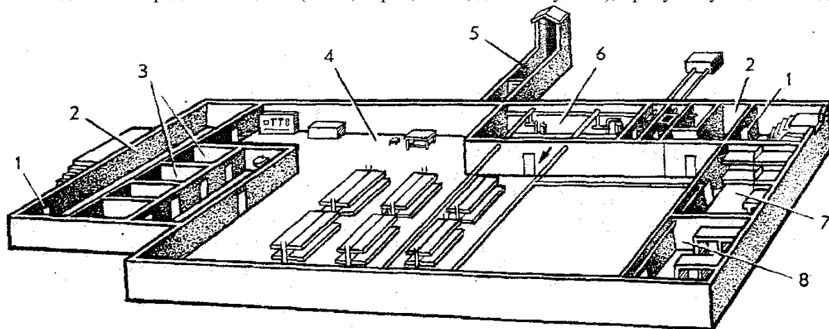
Рисунок 2.1 – План убежища
