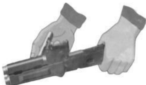
Рис. 7.17. Отделить затвор от затворной рамы
